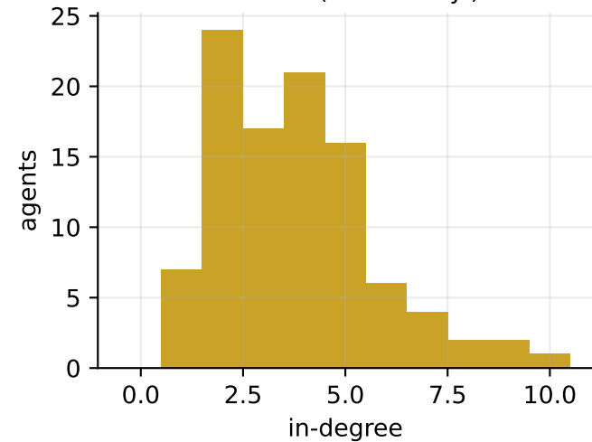
Random (Erdos-Renyi)
